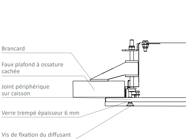
Montage encastré au plafond (LO)
