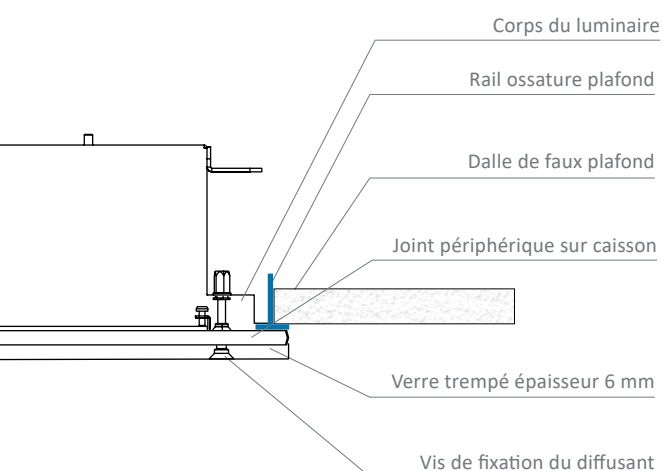
Montage sur plafond modulaire à ossature apparente (LI)
