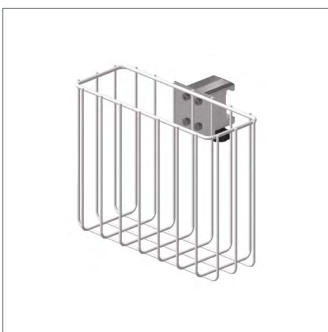
Panier en acier thermolaqué 250 x 90 x 200 mm avec pince pour rail horizontal Réf : 519162
