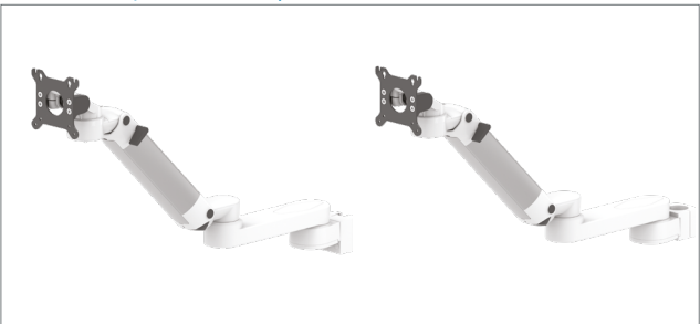
Bras ajustable en hauteur déport de 450 mm, débattement vertical 438 mm avec allonge de 230 mm pour écran VESA (max 16 kg)
