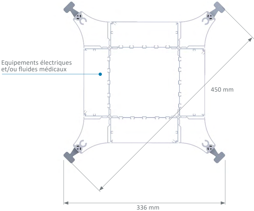
Vue en coupe (couvercle 160 mm)
