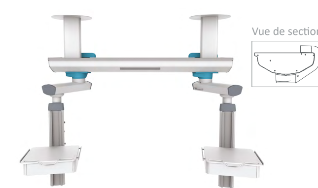
Configuration poutre HI-CARE avec boitier horizontal et nacelle.
