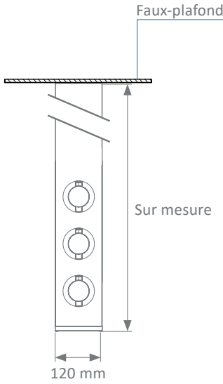
Boitier sans habillage
