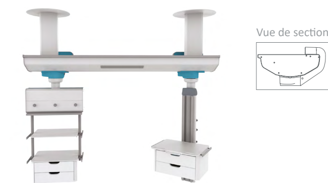
Configuration poutre HI-CARE avec boitier horizontal et boitier vertical.
