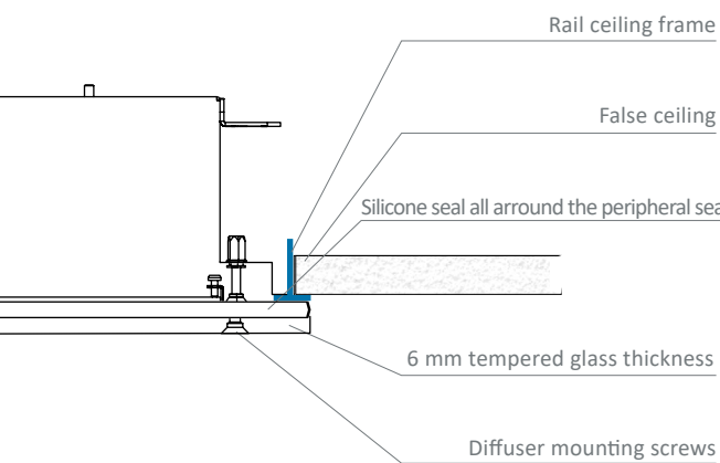
Lay-In (LI)
