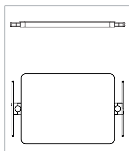
Plateau 605x455 mm avec rail latéraux (50 kg max)
