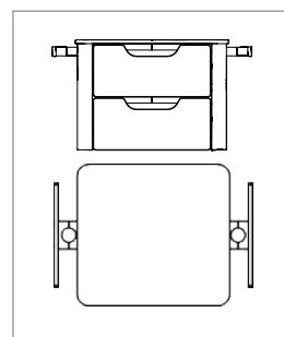
Bloc plateau 405x375 mm avec tiroir double et rails latéraux (40 kg max)
