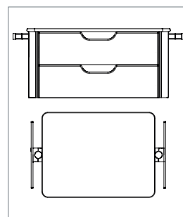
Bloc plateau 605x455 mm avec tiroir double et rails latéraux (50 kg max)*
