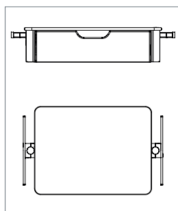
Bloc plateau 605x455 mm avec tiroir simple et rails latéraux (50 kg max)*
